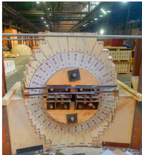
Стендовая сборка арки штуцера горячего дутья для АО «КМЗ».
