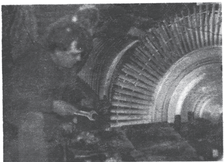
В турбинном цехе ЦЭС идет ремонт турбины мощностью 6 мВт.
